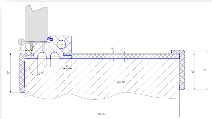
Схема установки с телескопическим наличником
