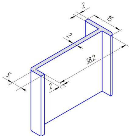
Алюминиевая притворная планка
